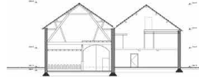
doorsnede B-B
